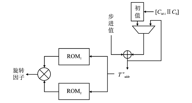
图 7 旋转因子生成单元
