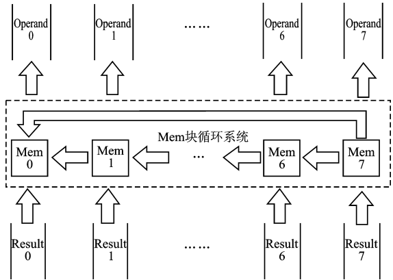
图 5 计算过程中存储块循环
