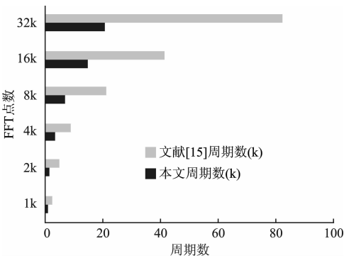
图 9 FFT 计算时间
