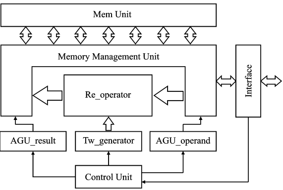
图 2 FFT 处理器结构框图
