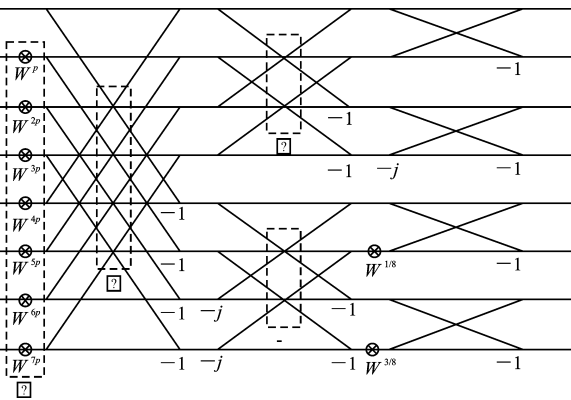
图 1 基 8 DIT-FFT 蝶形运算图
